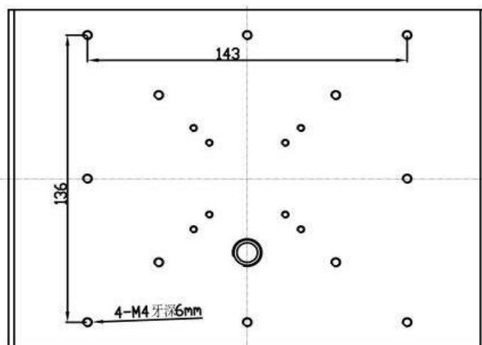
反光杯固定孔位：
